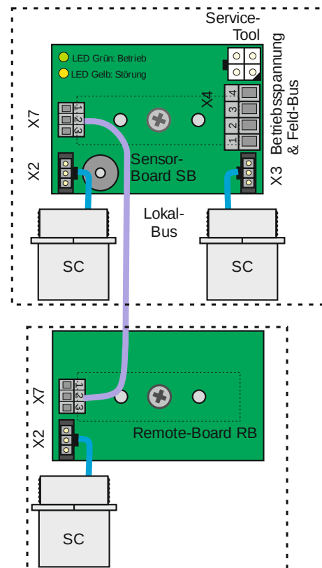
Abbildung 2: Sensor-Board SB mit 2 Sensoren und mit Option Remote-Board RB mit 1 Sensor
